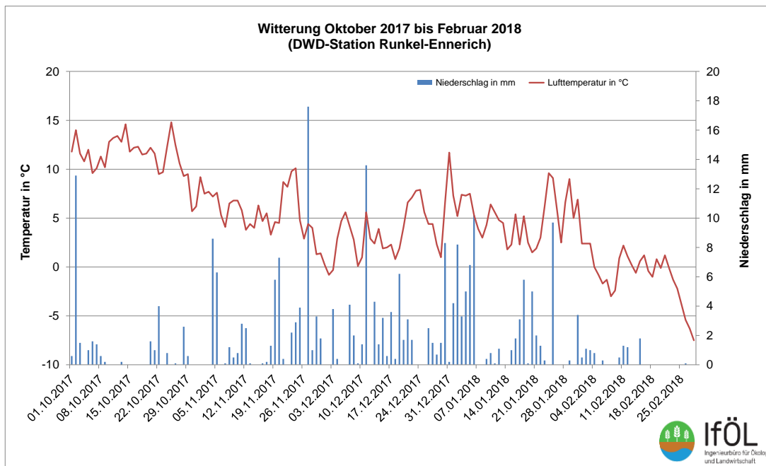
Abbildung 1: Temperatur und Niederschlag von Oktober 2017 bis Februar 2018 (DWD-Wetterstation Runkel-Ennerich).
